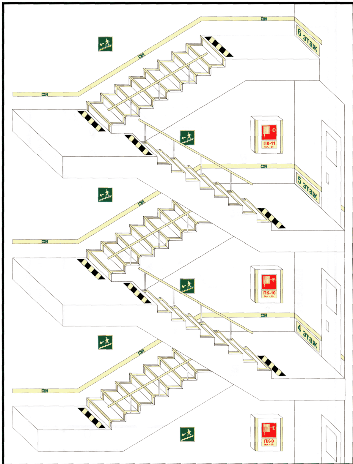
Рисунок Б.5 - Пример размещения элементов ФЭС на лестницах
